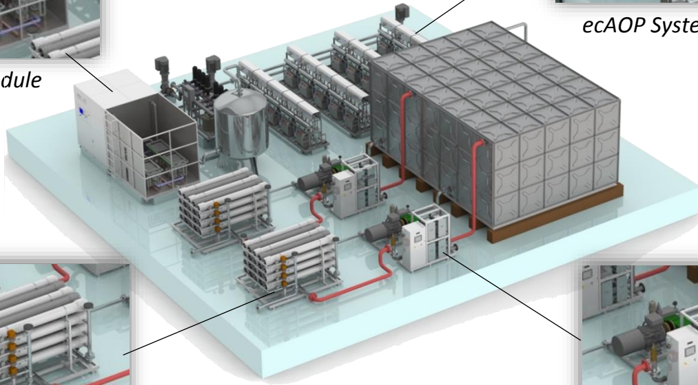
RO Module ( TORAY membrane)
